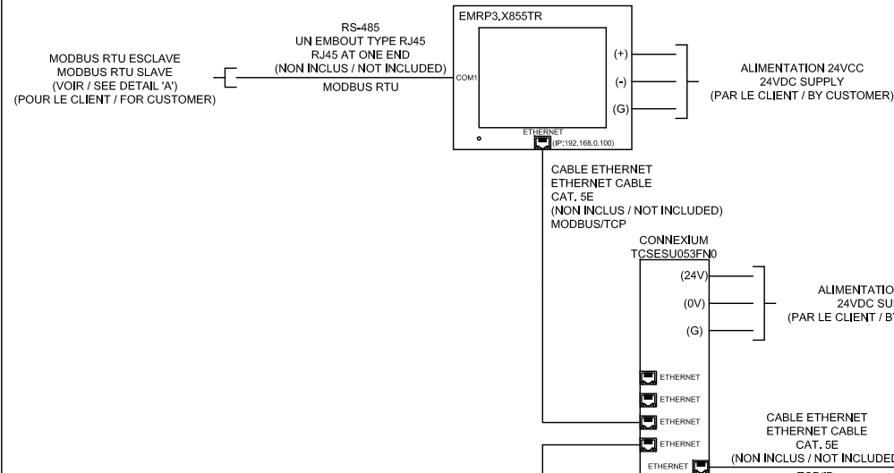
EMRP3.X855TR CONFIGURATION OPTIONNELLE OPTIONAL SETUP
