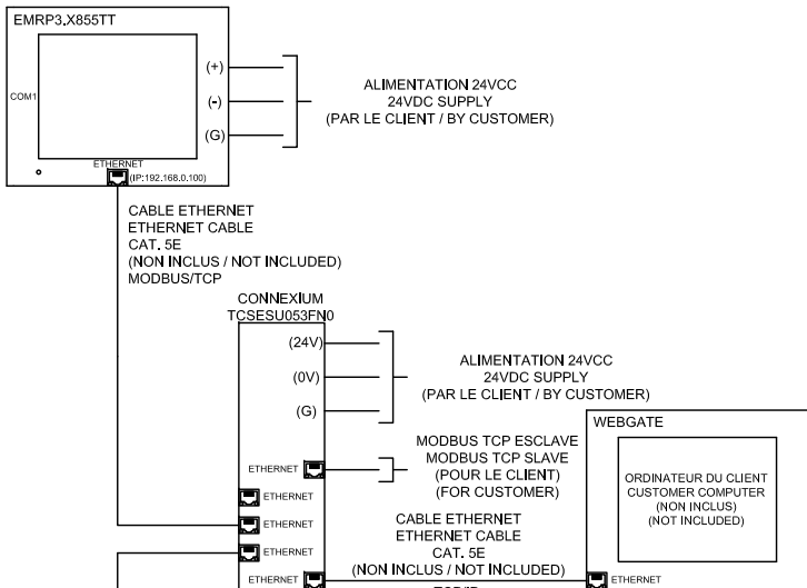
EMRP3.X855TT CONFIGURATION OPTIONNELLE OPTIONAL SETUP
